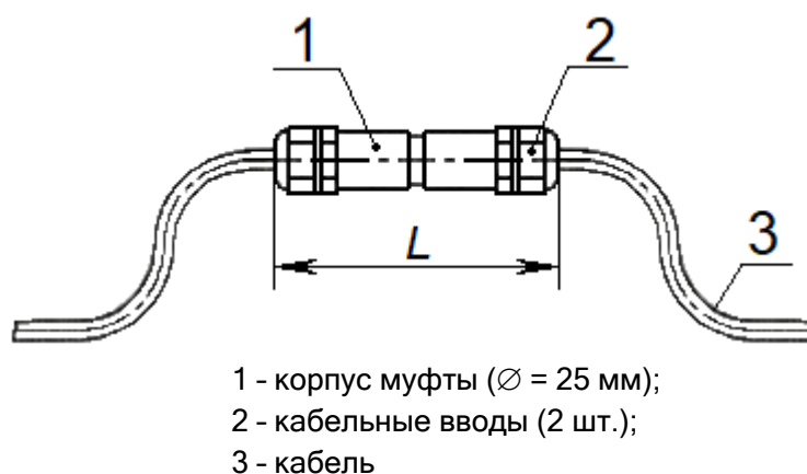
Рисунок 1 - Общий вид муфты
